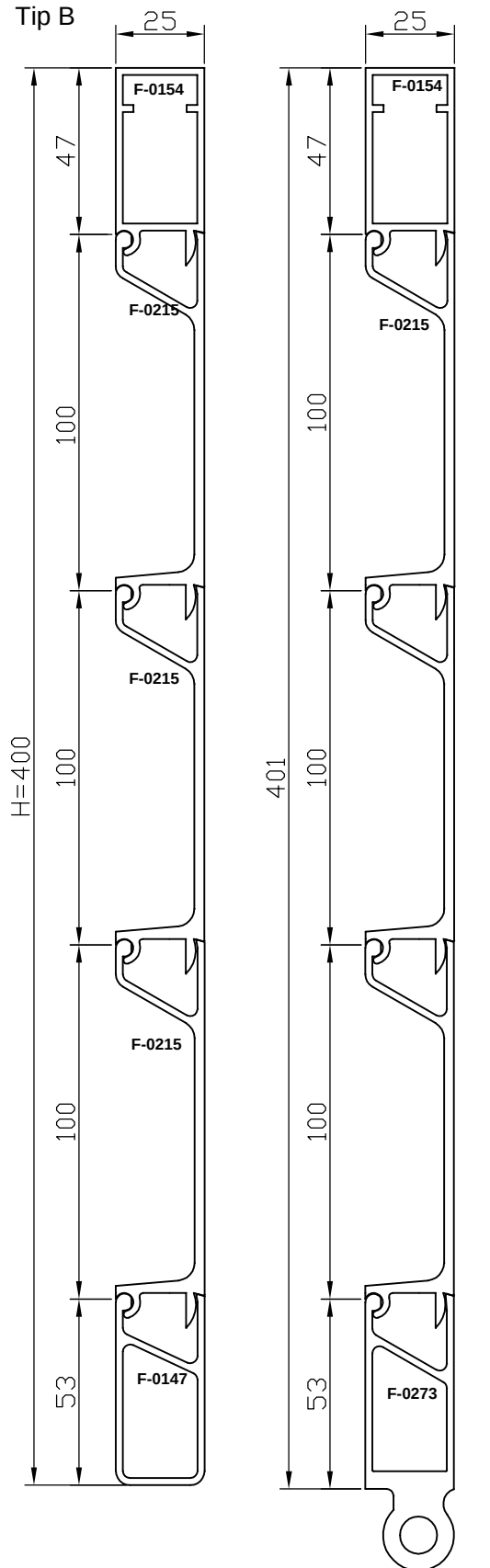
PRESJEK 1-1
