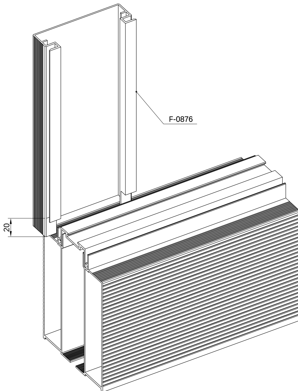
POGLED A-A
