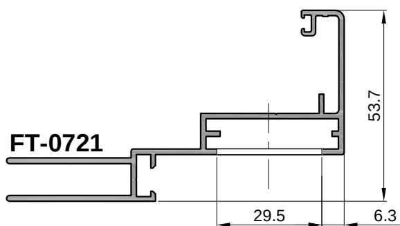
PRESJEK 1-1
