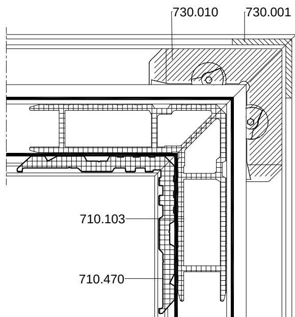
PRESJEK B-B
