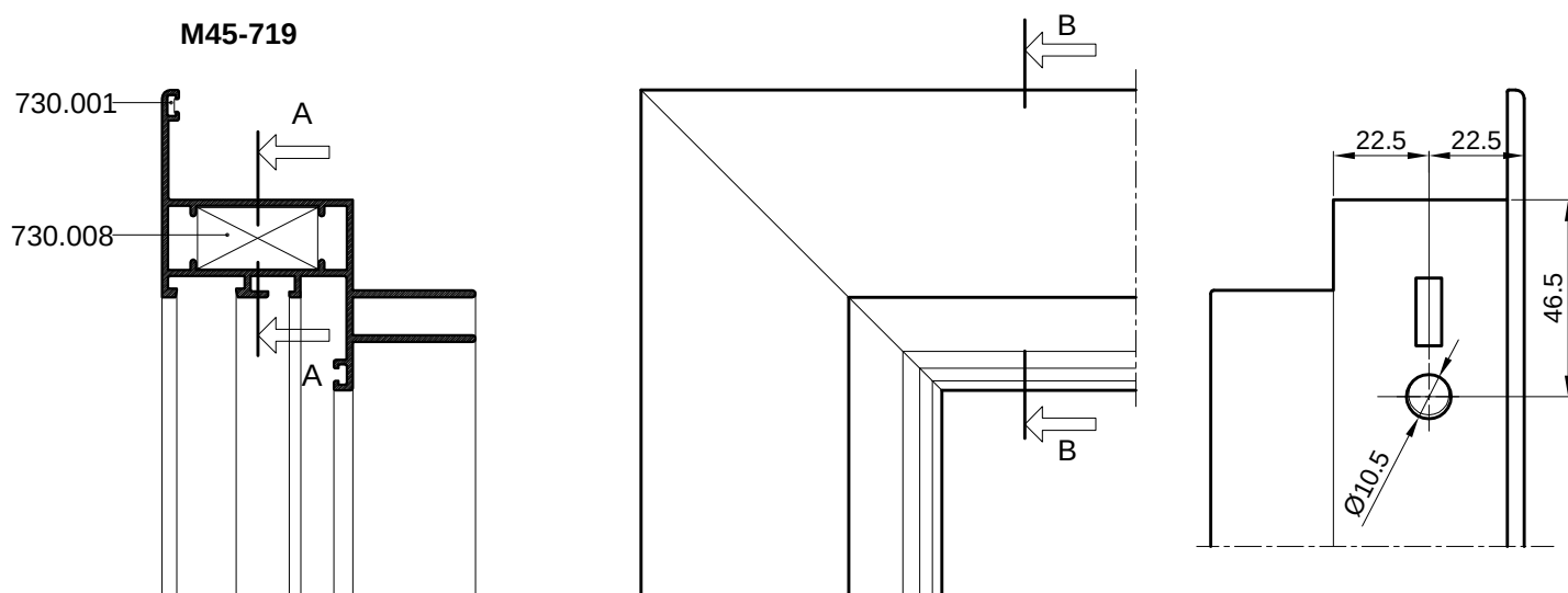
PRESJEK B-B
