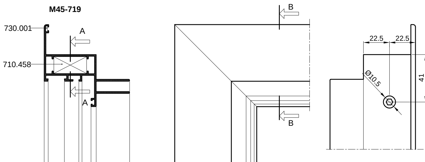
PRESJEK B-B
