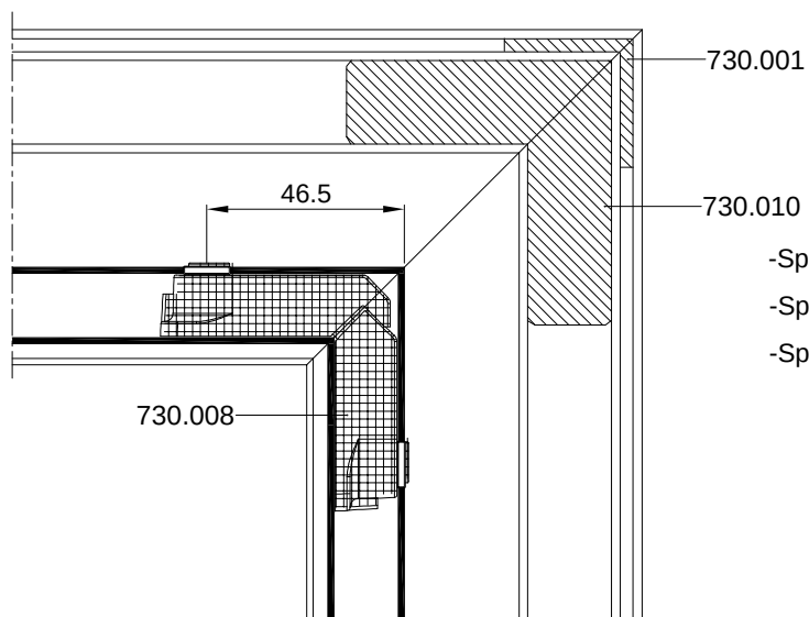
PRESJEK A-A
