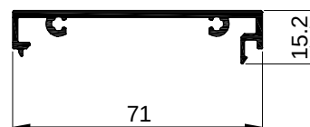
F-1667 M 1:2
