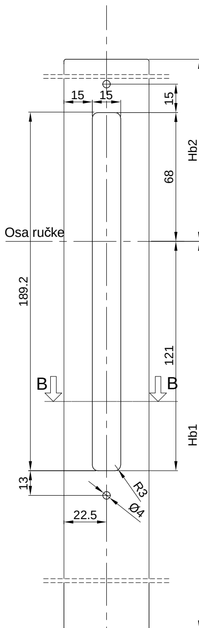
Presjek B-B M 1:2 F-1659
