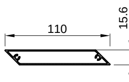
F-1663 kg/m 0,823
