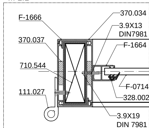
Detalj A M 1:1
