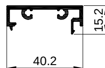
F-1660 M 1:2
