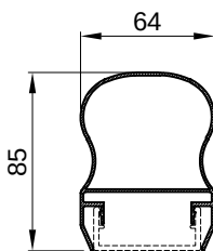
F-1334 kg/m 1.185
