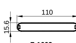
F-1662 kg/m 0,83
