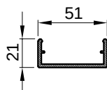
F-0620 kg/m 0.600
