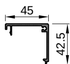
F-1659 kg/m 0,517
