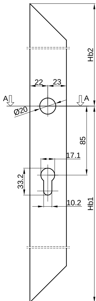
PRESJEK A-A M 1:2
