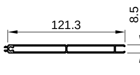
F-0714 kg/m 0,895
