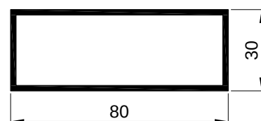
F-0441 M 1:2
