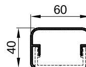
F-0689 kg/m 0.740
