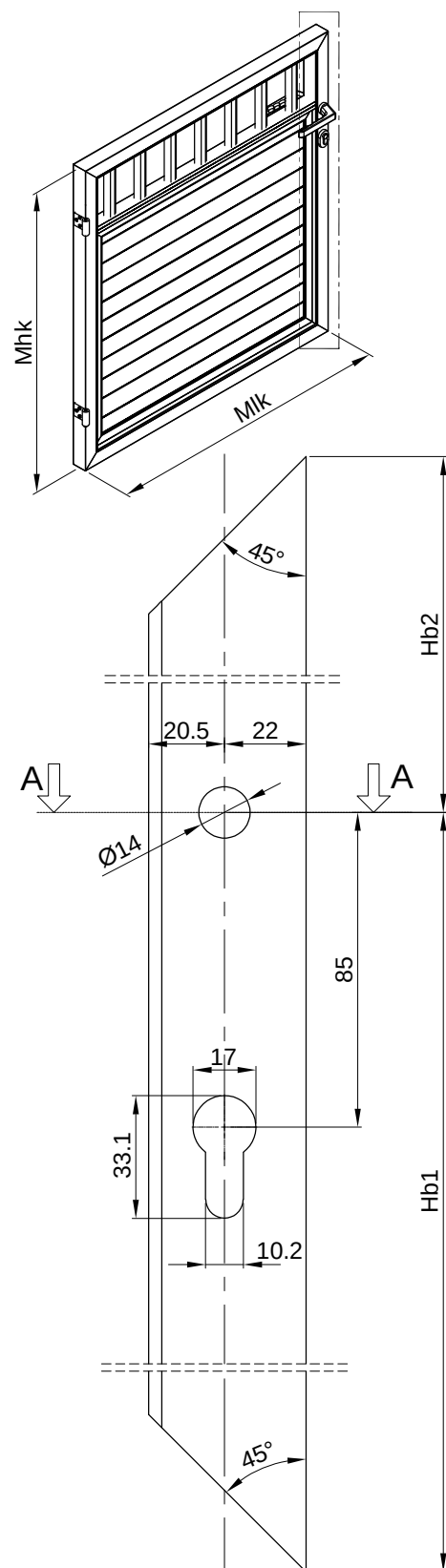
Presjek A-A M 1:2 F-1659
