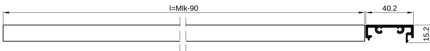
Presjek A-A M1:2 F-1660
