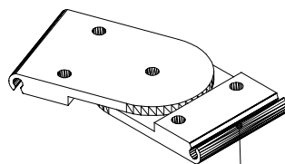
521.051 Veznik sa promjenljivim kutom Vijak M6x8 DIN 913
