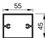
F-0356 kg/m 1,06
