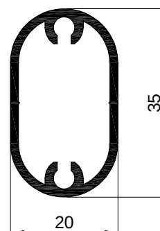
OG-111 M 1:1
