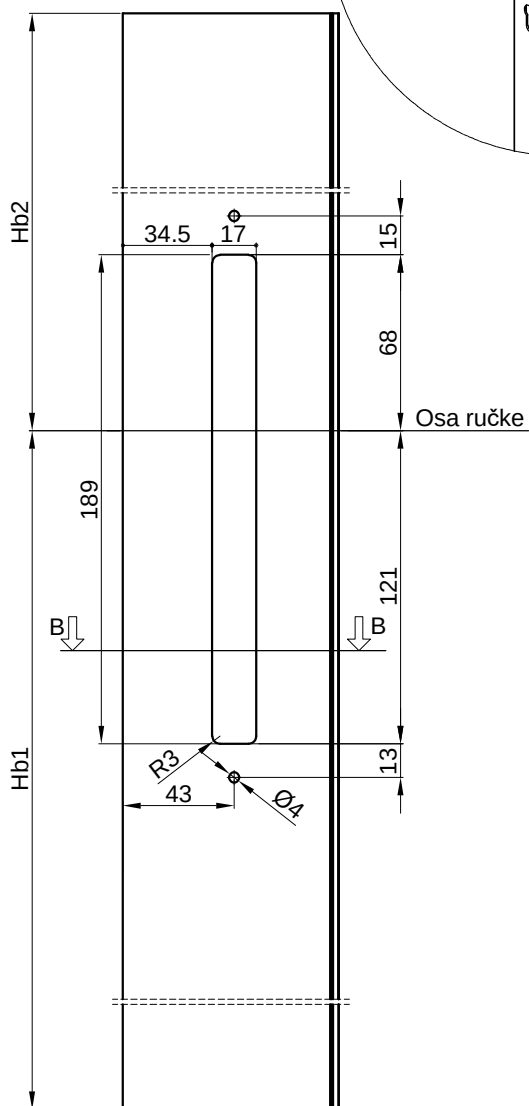
PRESJEK B-B M 1:2
